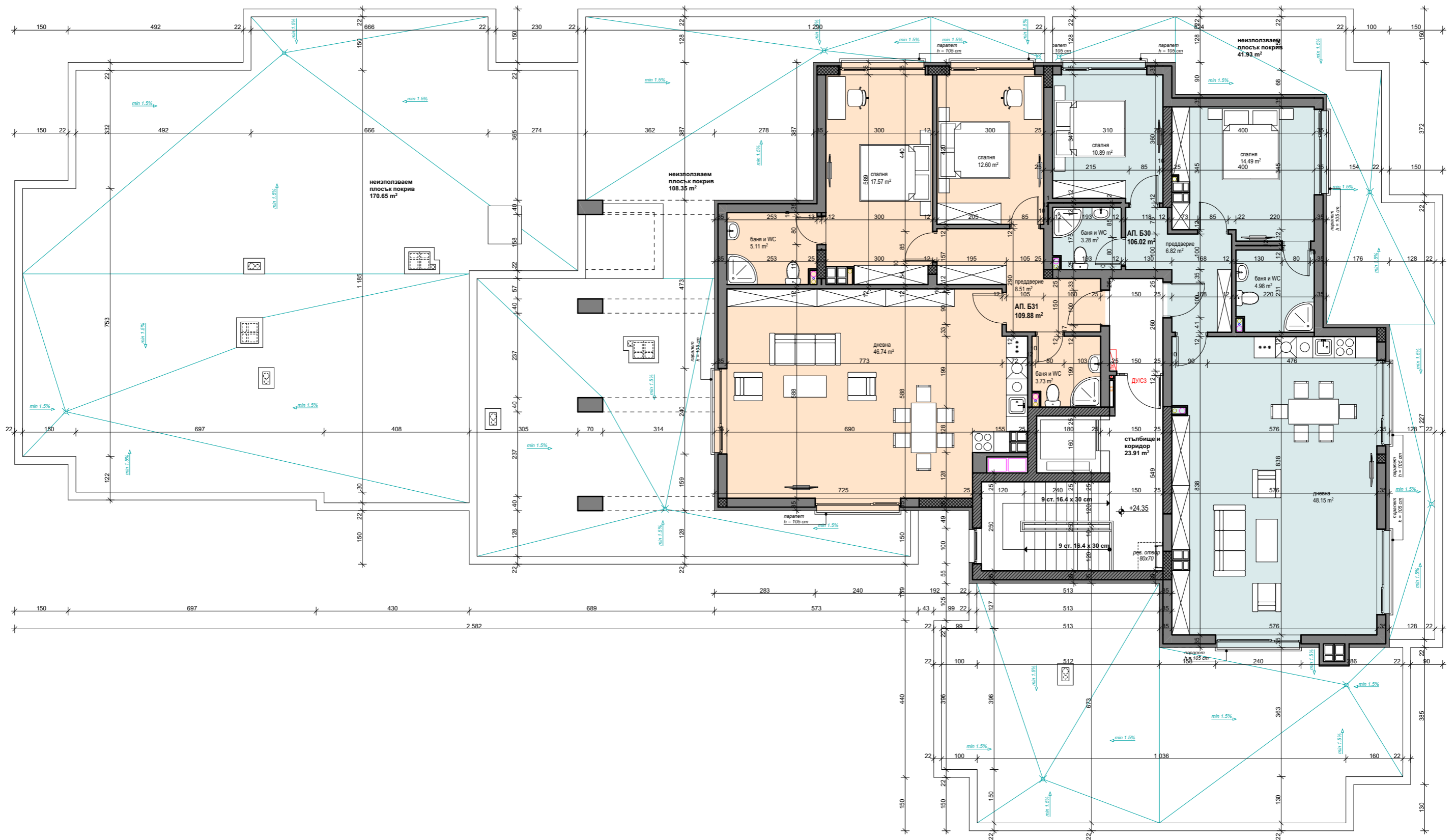
РАЗПРЕДЕЛЕНИЕ кота +24.35 /девети етаж/
