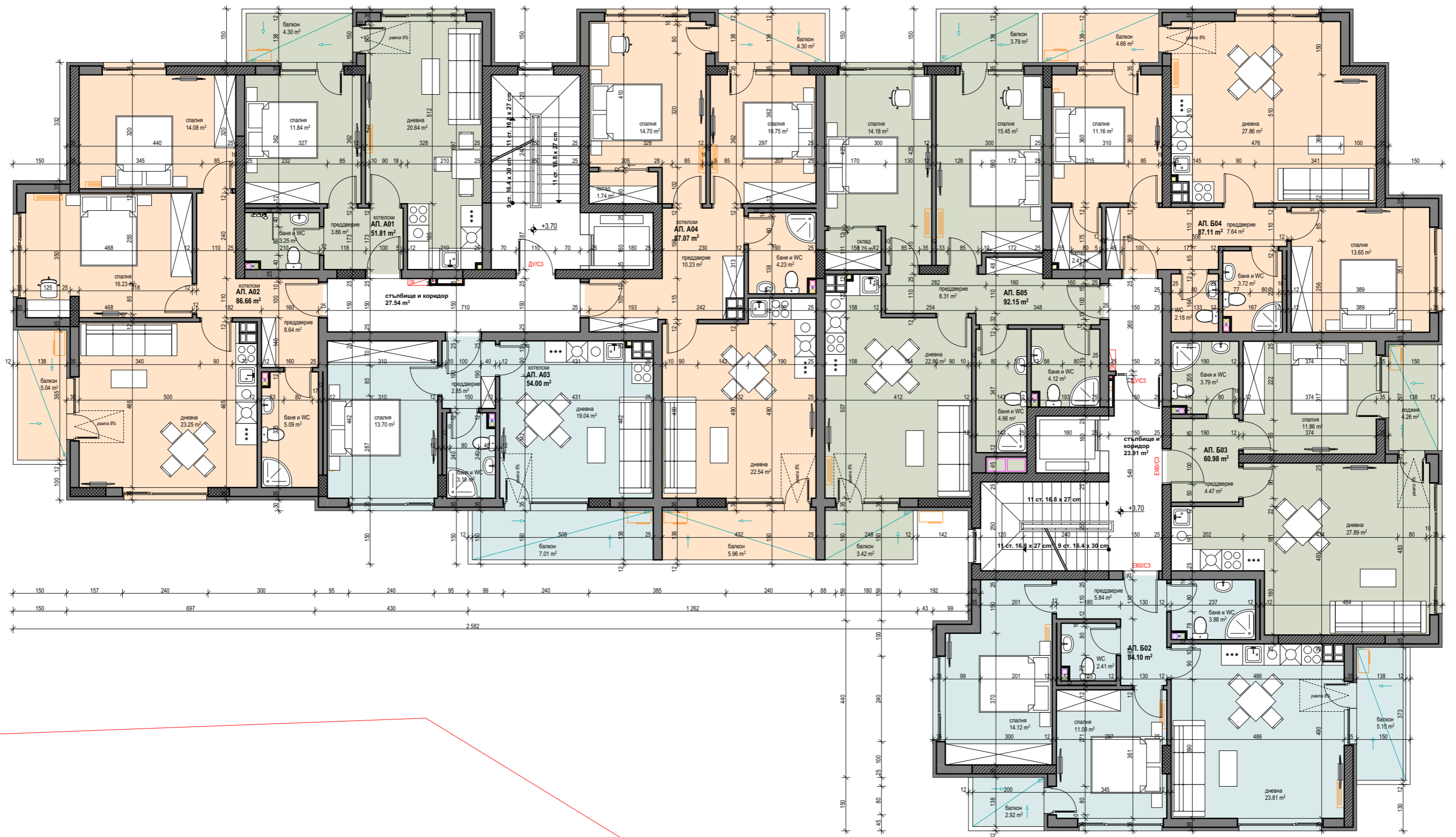
РАЗПРЕДЕЛЕНИЕ этажа +3.70 / втори етаж/
