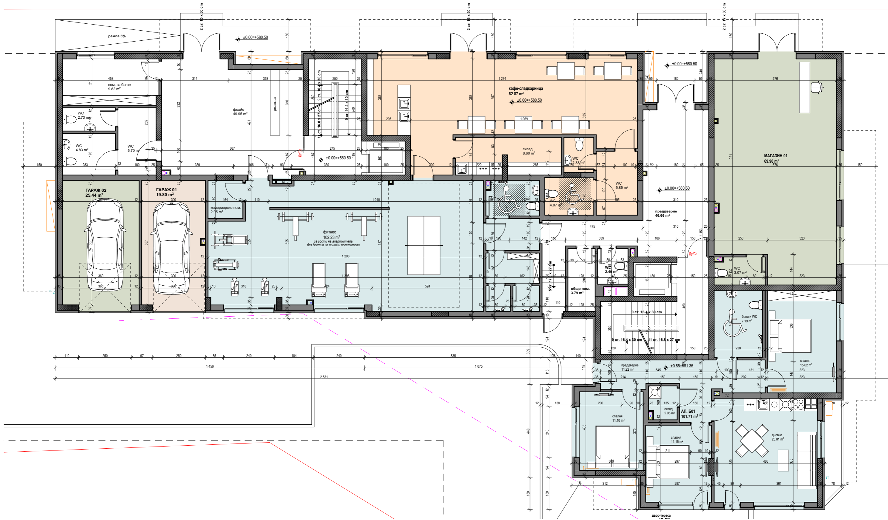
РАЗПРЕДЕЛЕНИЕ кота ±0.00 /първи етаж/
